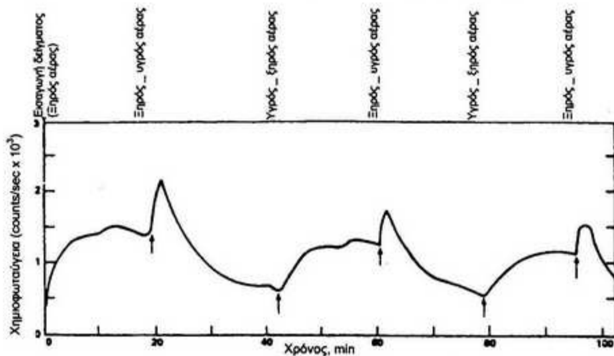
Εικόνα 1: Αποτέλεσμα της κυκλικής μεταβολής της υγρασίας στους 70°C στην χημιοφωταύγεια του χαρτιού (Πηγή: Fellers κ.ά., 1989, σελ. 61, σχ. 4.4.).
