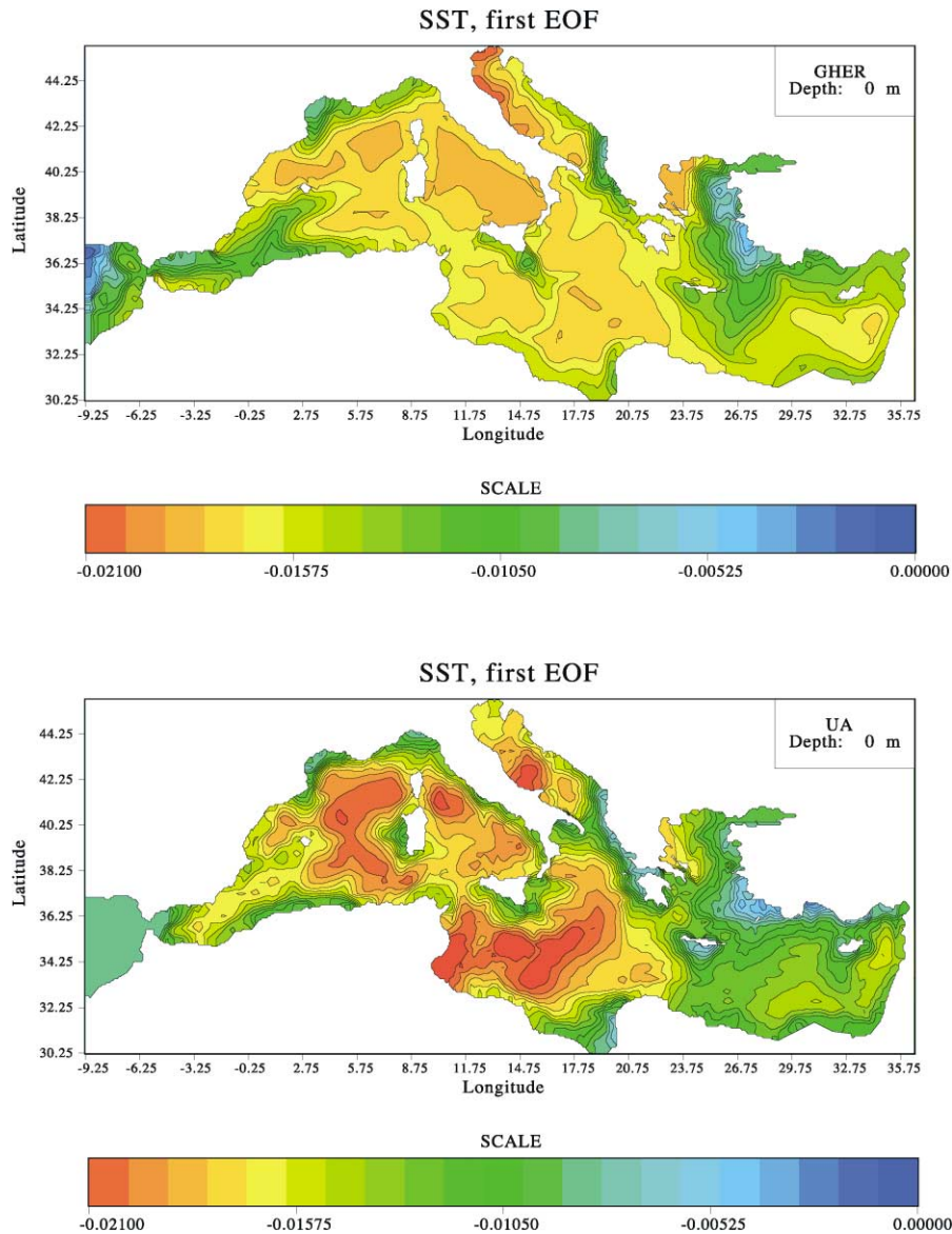
Fig. 20. First SST EOF.
